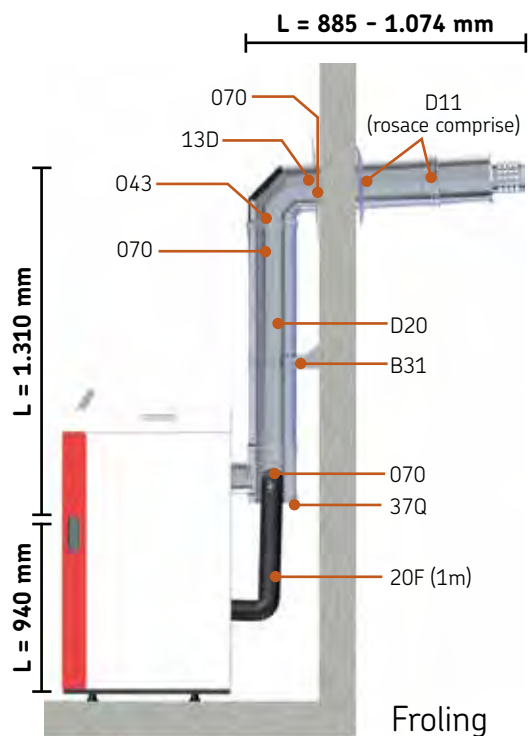
KIT HORIZONTAL POUR CHAUDIÈRE FRÖLING SORTIE ARRIÈRE Ø 130/200 INOX
