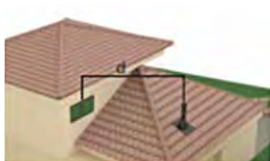
F Distance à un pignon de la même habitation. d > 4 m. d > 1 m en l'absence d'ouvrant ou d'entrée d'air.
