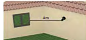
D Par rapport à un angle rentrant, zone d'interdiction avec un mur adjacent contigu à un ouvrant.
