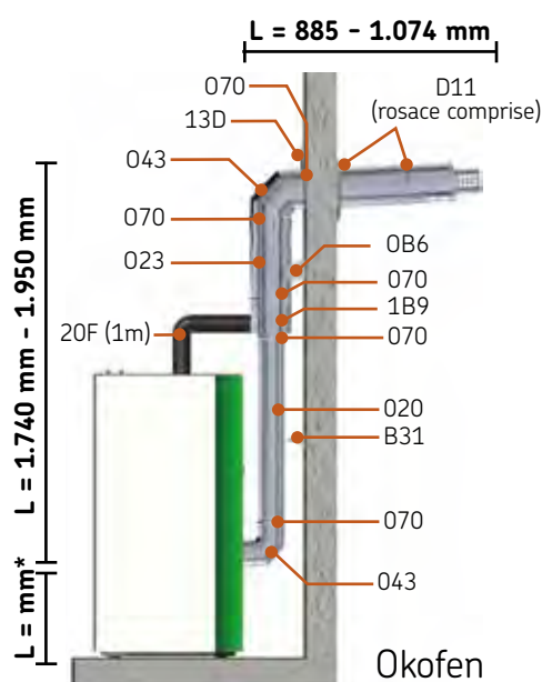
KIT HORIZONTAL POUR CHAUDIÈRE OKOFEN CONDENSATION Ø 130/200 INOX
