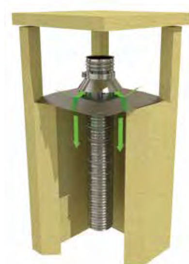
plaque étanchéité pour chapeau béton
